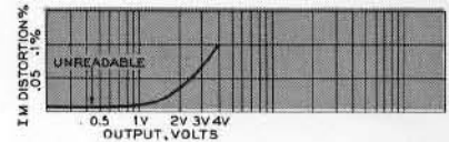
IM distortion.
