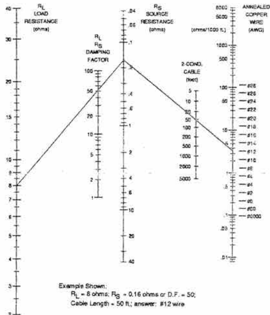
Fig. A.4 Wire-Size Nomograph
