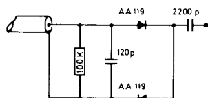
Fig. 3. Diodeprobe.
